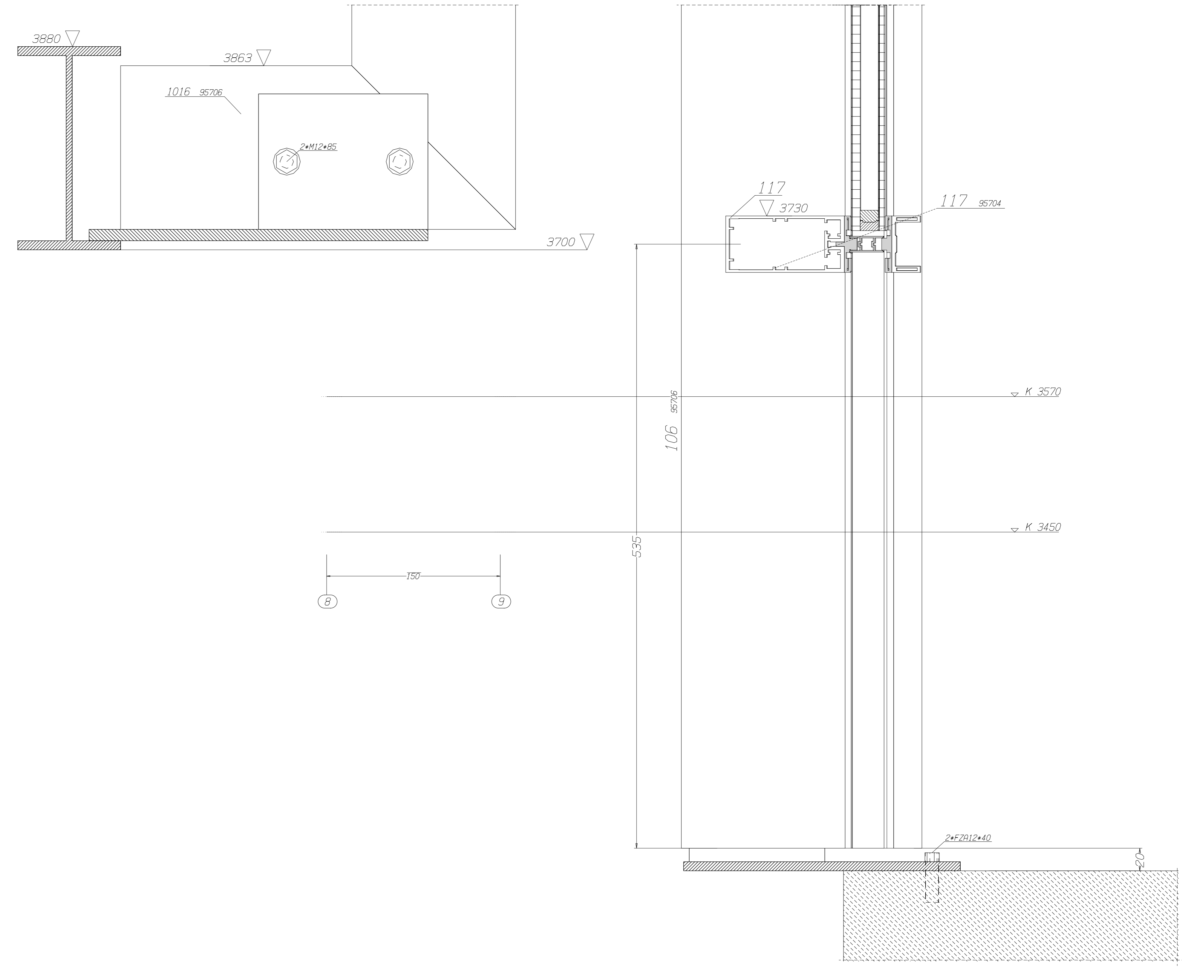
Vertikalschnitte Maßstab 1:2
